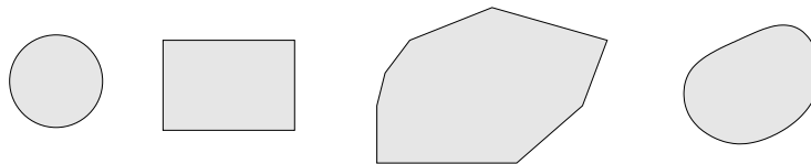
Figur 5.1: Några konvexa mängder
