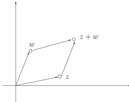
Figur 1.1: Geometrisk tolkning av z + w .
