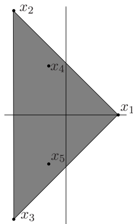
Figur 5.5: Rötterna till polynomet x^3 + x^2 + 3x - 5 och dess derivata
