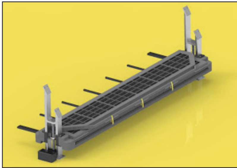
Infällt läge - Reglar infällda och fastspända
