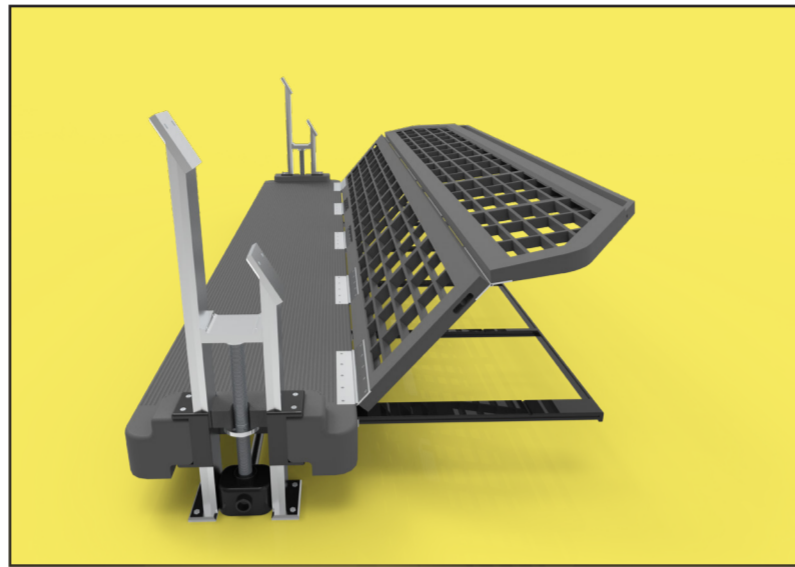
Reglar skjuts ut och plattformen fälls
