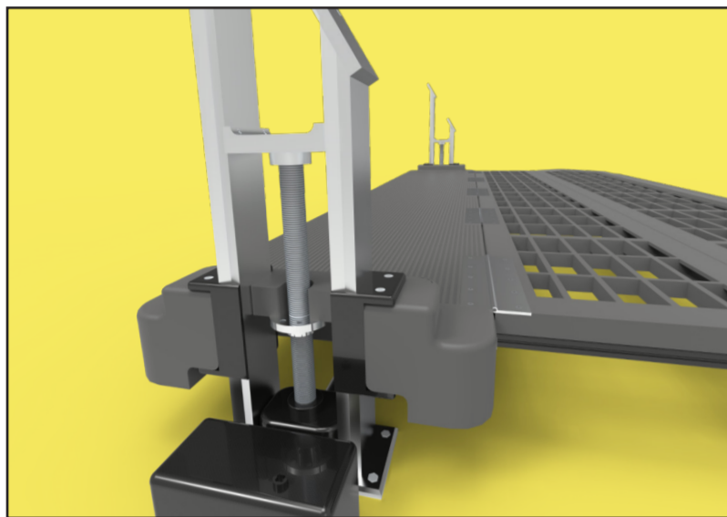
Gejdersystem, motor samt skruvdomkraft som hissar
