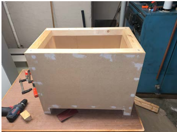
Bild 26: Ihopsättning av stomme.
