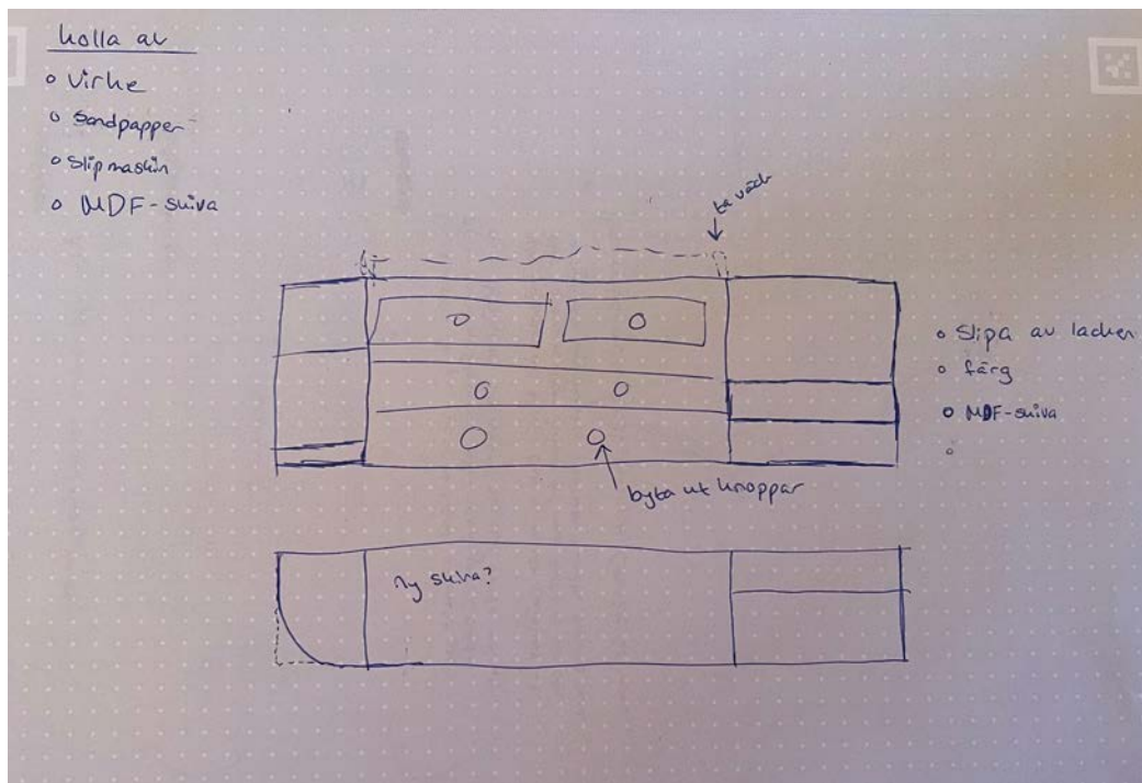
Bild 5: Första idéskissen av byrån där dekoreringslisterna var kapade, vänstra sida med en rundad hylla samt höger sida med en sittdel.
