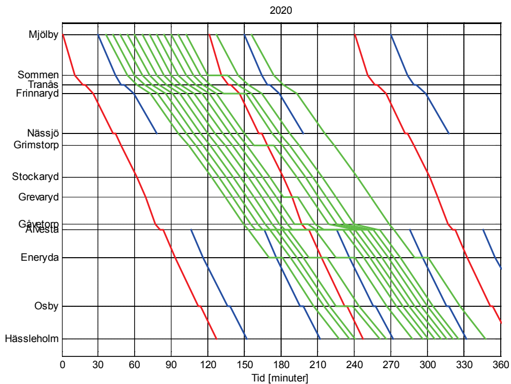
Figur 20. Exempel på tidtabell med 2020 års persontrafikintensitet. Röda streck är snabbtåg Stockholm–Malmö, blåa interregio- och regionaltrafik, och gröna streck är godståg. I detta exempel ryms 13 godståg på två timmar, det vill säga 6,5 godståg/timme.
