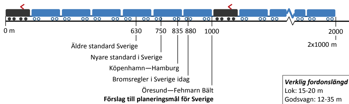
Figur 29. Möjliga godstågslängder i Sverige och Köpenhamn–Hamburg.
