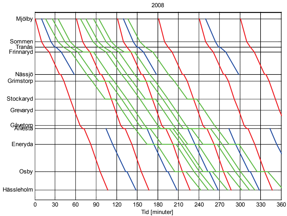
Figur 19. visar ett exempel på tidtabell med 2008 års persontrafikintensitet. Röda streck är snabbtåg Stockholm–Malmö, blå interregio- och regionaltåg och gröna streck godståg. I detta exempel ryms 7 godståg på två timmar, det vill säga 3,5 godståg/timme.
