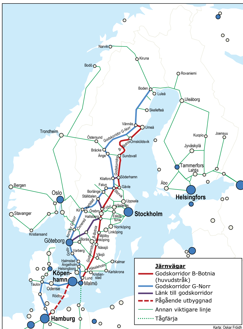
Figur 21. Godskorridorerna B–Botnia (huvudstråk) och G–Norr i analysen.
