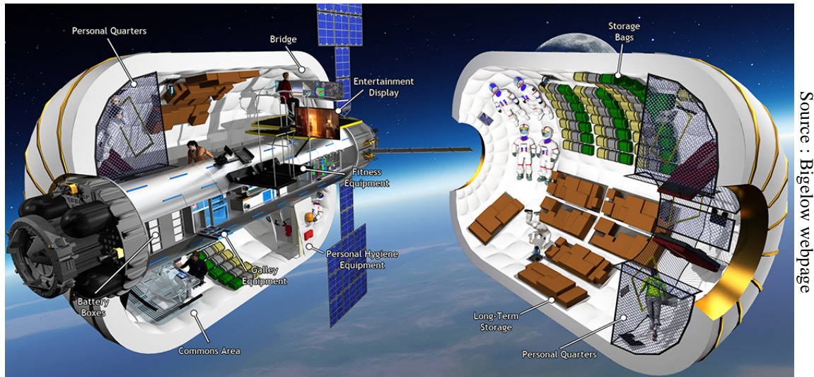
Fig.11 BA 330
