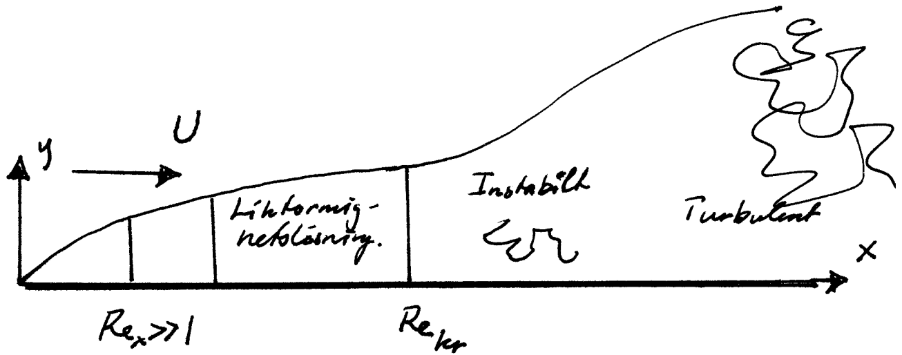
Figure 3: De olika stadierna i gränsskiktets utveckling. Först då Re_x \gg 1 börjar gränsskiktsapproximationen att gälla. Därefter så kommer så småning Blasiuss likformighetslösning att gälla. Vid Re_x = Re_{kr} \approx 5 \times 10^5 blir gränsskiktet instabilt och en bit nedströms blir det fullt turbulent.
