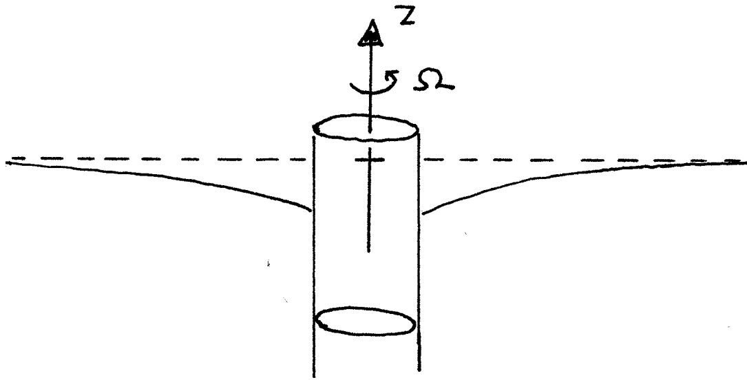
Figure 1: En roterande cylinder som är nedsänkt i vatten genererar en virvel omkring sig i vattnet. I en virvel sjunker trycket mot centrum. Därför kommer den omgivande vattenytan att sjunka kring cylindern.
